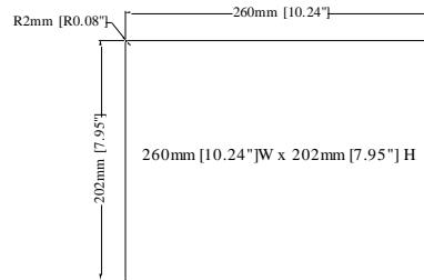
Cutout Dimensions
